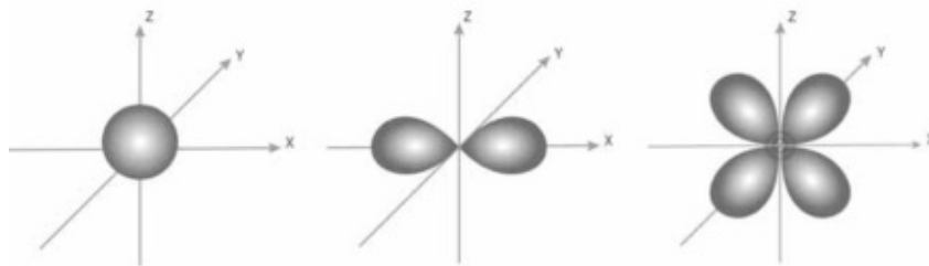
Рисунок 3. Различные формы электронного облака («геометрия» квантовой химии):
