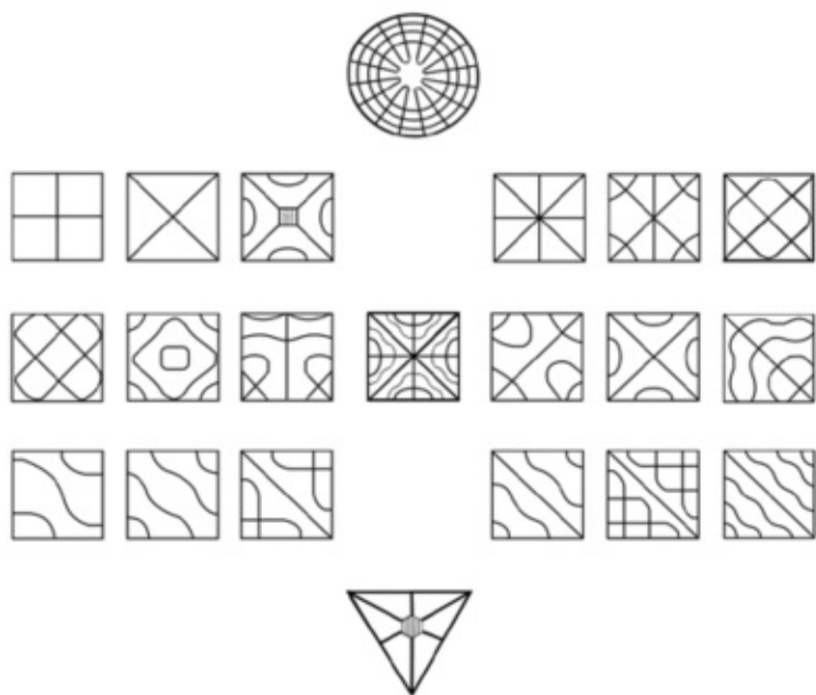
Рисунок 63. Фигуры Хладни.
