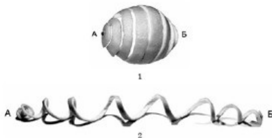
Рисунок 4. Образный пример преобразования электрона из частицы в волну:
